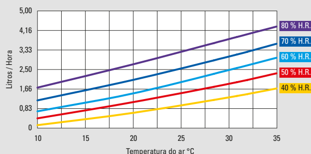
Capacidade de desumidificação DS 60
