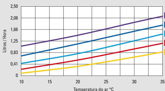
Capacidade de desumidificação DS 30
